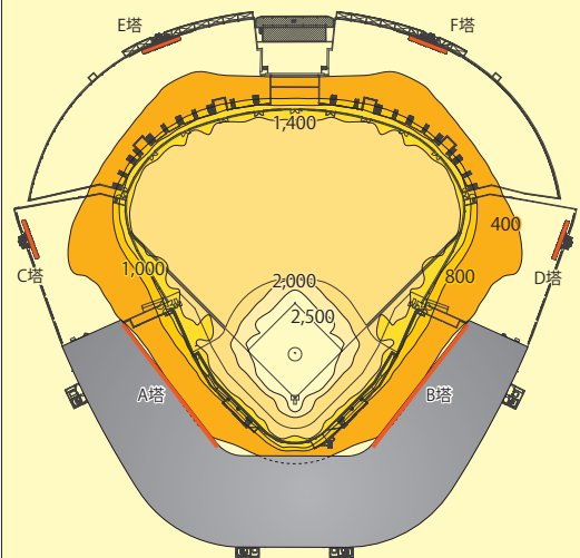
設計値 全点灯パターン（プロ野球時）
