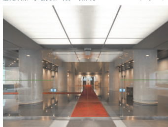
議会棟・事務棟風除室には直管形LEDベースライト1灯用器具を設置
