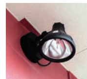
壁面下方を照射している150Wセラミックメタルハライドランプ投光器
