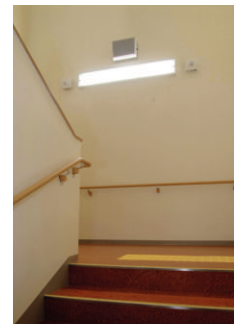
階段の人感センサー対応階段灯調光タイプ 灯具の横に人感センサーを設け、人を感じて100%点灯、人がいないときは25%に減光
