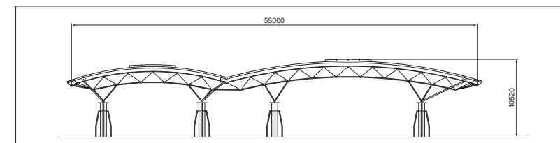
大屋根の立面図
