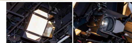
(左) LEDブロードライト(バンドア鏡面仕様)① (右) LEDスポットライトFORTEX8型フレネル②
