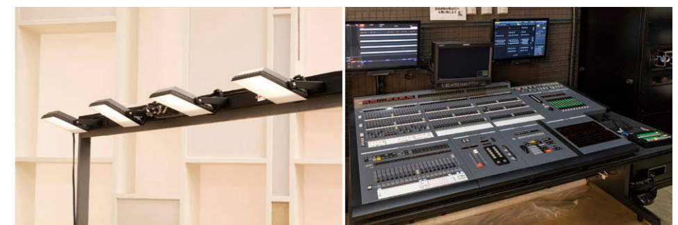
小形投光器によるライティング 主役である商品をより美しく撮影するため一部LED小形投光器④を活用。 調光操作卓 ジュピターショップチャンネル仕様とした調光操作卓⑦
