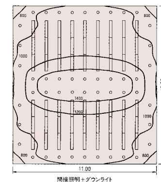
照度分布図
