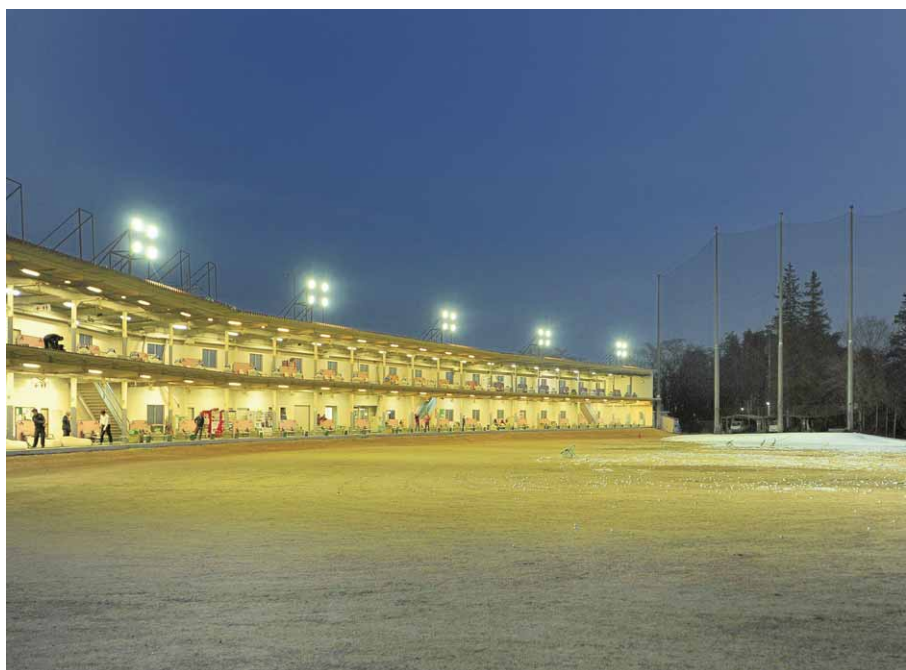
屋根上に照明やぐらを4基設け、1基当たりLED投光器を4台設置。細かに照射角度を調整し、滑らかな水平照度と空間照度も高めてボールの球筋がよく見える光環境を確保
